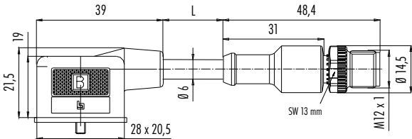
Verbindungsleitung Magnetventilsteckdose – Kabelstecker M12
