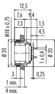
Flanschdose mit flexibler Leiterplatte, von vorn verschraubbar
